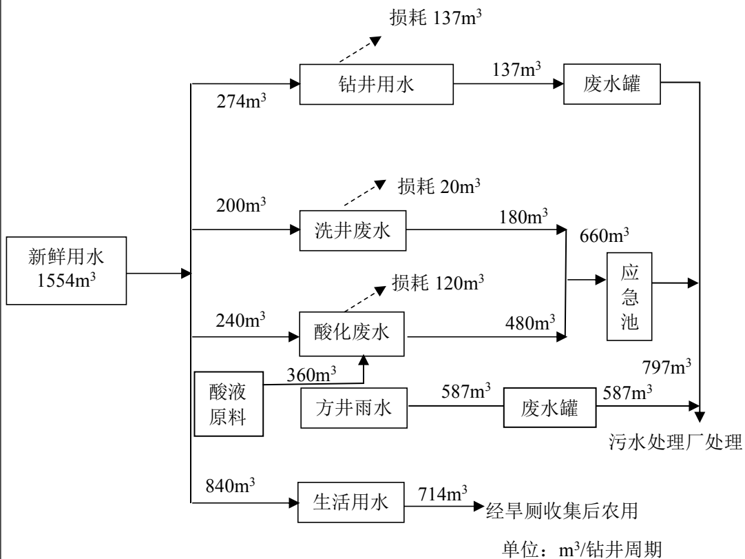
图 4.3-5 磨溪 039-H1 井钻井水平衡图
