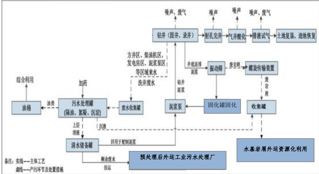
图 4.3-1 钻井工程井场污染物走向流程示意图
