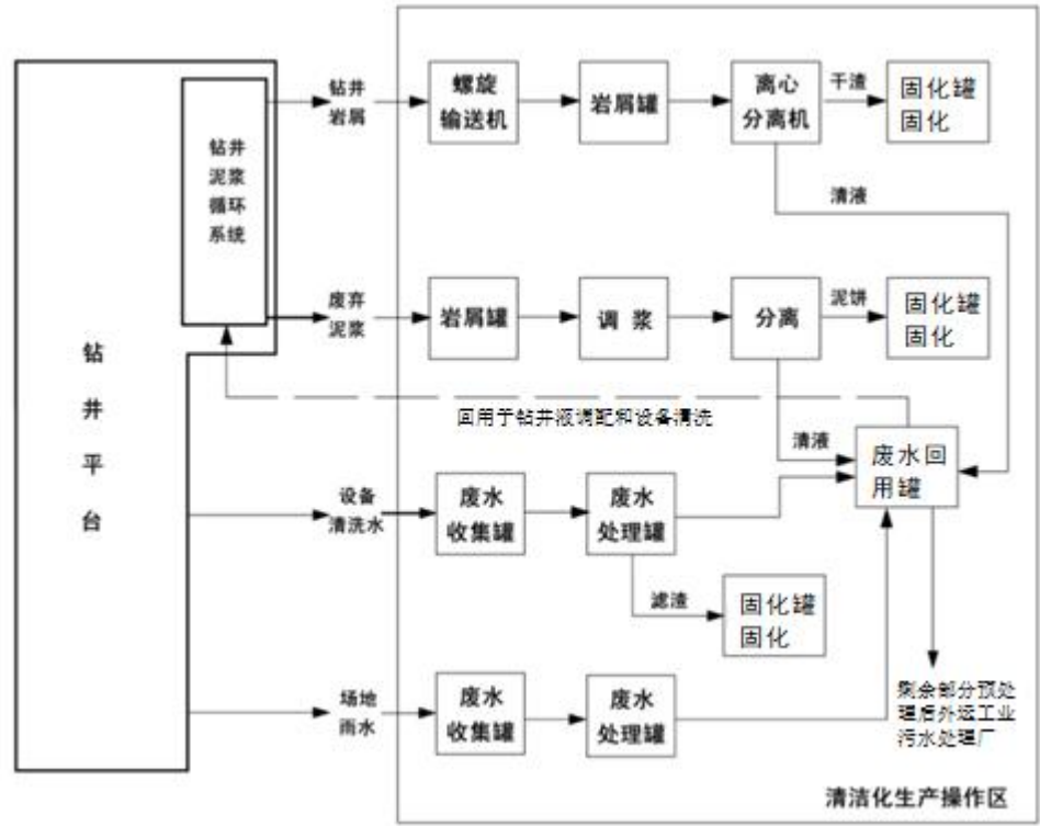
图2.11-4 清洁化操作方案流程图
